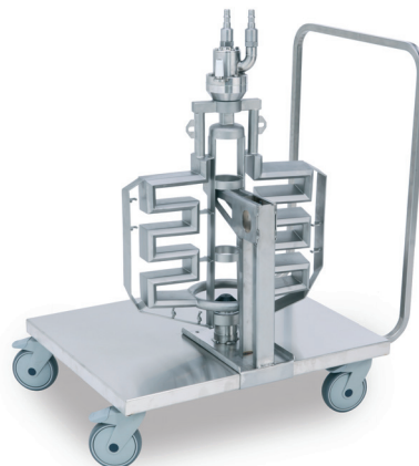
Vozík na mytí míchadla MWT
